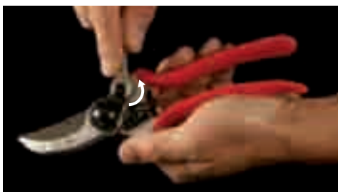
4. Desmontar la hoja, y si fuera necesario, cambiarla por otra
